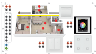
Panel UV-139, INELS chytrá domácnost - BYT, demonstrační panel elektrických ovládacích prvků a spotřebičů v bytě.
